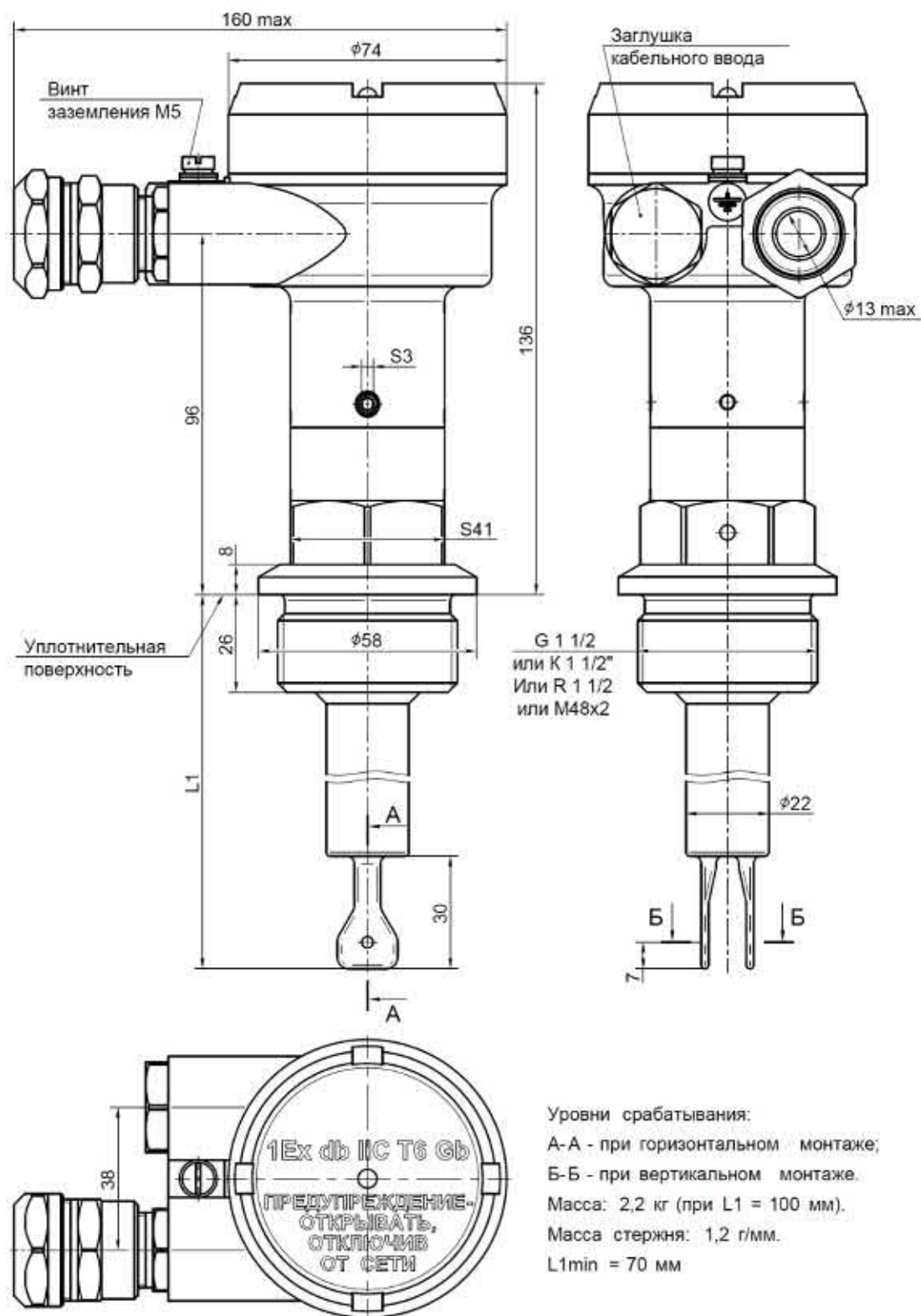
Рисунок Д.9 Габаритные и установочные размеры сигнализаторов со способом присоединения штуцер M48x2, G1 1/2 для работ при температурах контролируемой среды не более 100 °С (по специальному заказу возможно изготовление сигнализаторов для работы при температурах контролируемой среды до 160 °С в указанных габаритах) с корпусом блока электронного, изготовленным методом высокоточного литья из нержавеющей стали, и механизмом поворота блока электронного.
