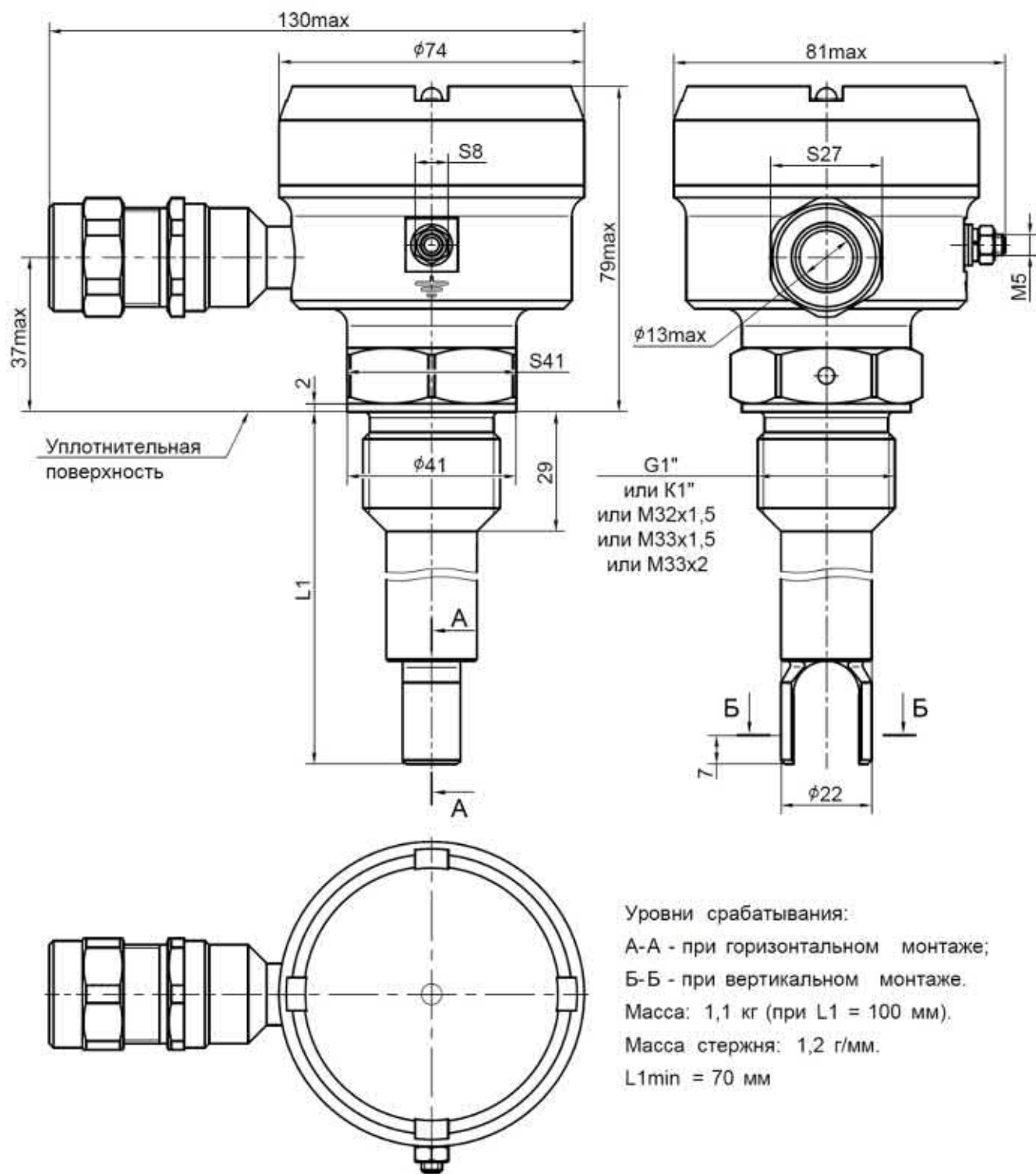
Рисунок Д.4 Габаритные и установочные размеры сигнализаторов со способом присоединения штуцер M32x1,5, M33x1,5, M33x2, G1, K1 для работ при температурах контролируемой среды не более 100 °С.
