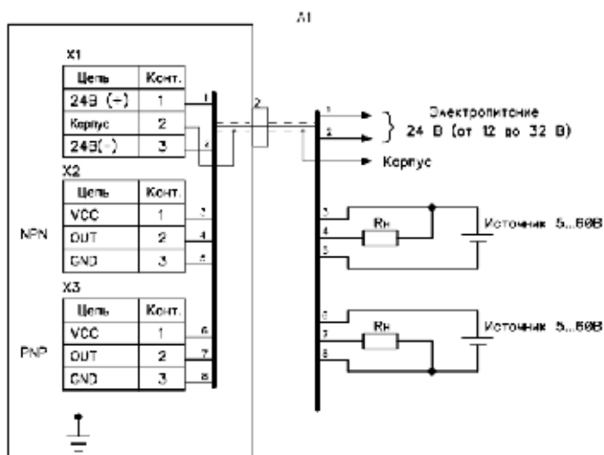
1.1.1.1 Рисунок Г.6 Схема электрическая подключения датчика исполнения TP
