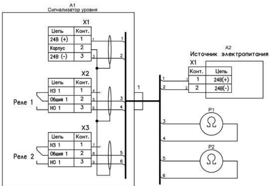
Рисунок И.2 Схема электрическая подключения сигнализатора исполнений Р1 и Р2 при проверке работоспособности
