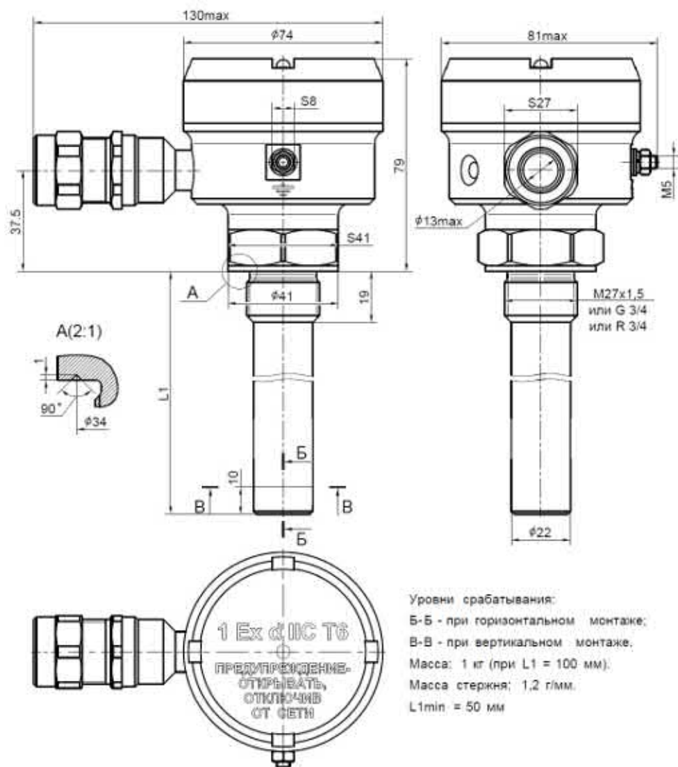
Рисунок Д.17 Габаритные и установочные размеры сигнализаторов со стержневым чувствительным элементом со способом присоединения штуцер M27x1,5, G3/4, R3/4 для работ при температурах контролируемой среды не более 100 °С.
