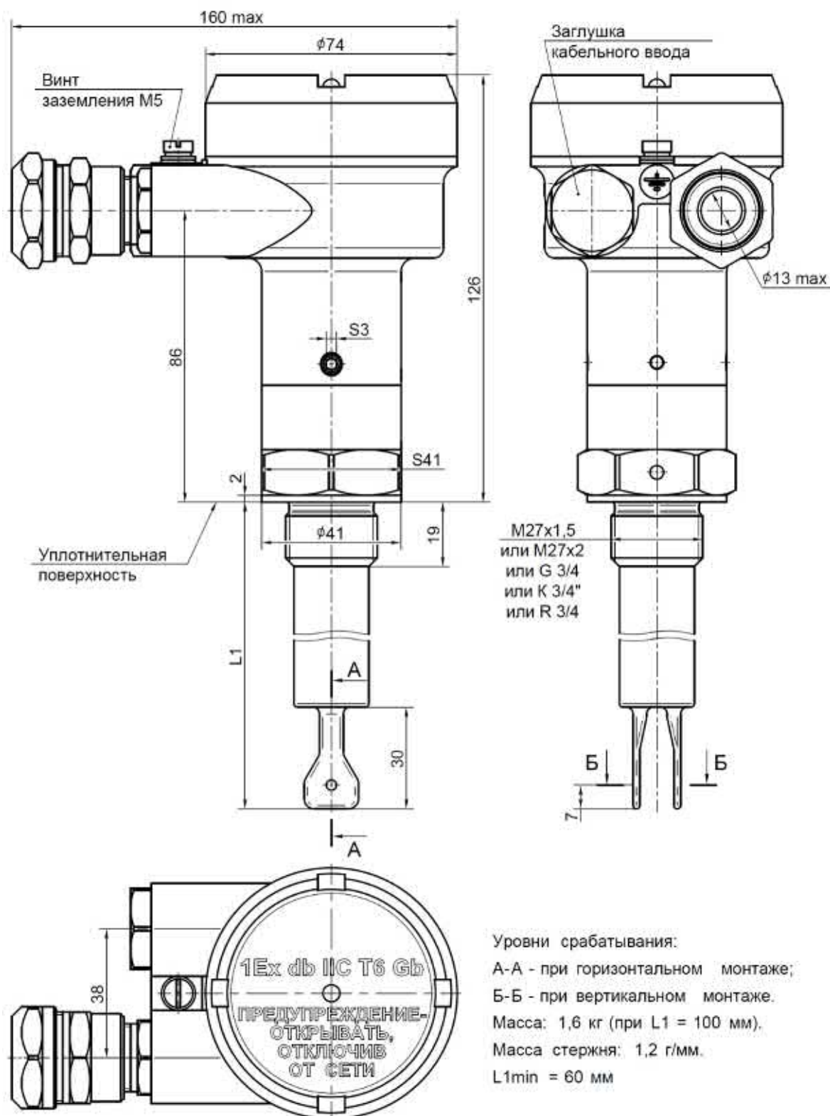
Рисунок Д.3 Габаритные и установочные размеры сигнализаторов со способом присоединения штуцер M27x1,5, M27x2, G3/4, K3/4 для работ при температурах контролируемой среды не более 100 °С (по специальному заказу возможно изготовление сигнализаторов для работы при температурах контролируемой среды до 160 °С в указанных габаритах) с корпусом блока электронного, изготовленным методом высокоточного литья из нержавеющей стали, и механизмом поворота блока электронного.
