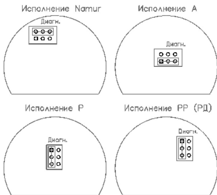
Рисунок 7. Положение переключки при переключении сигнализатора в режим «Настройка порога»
